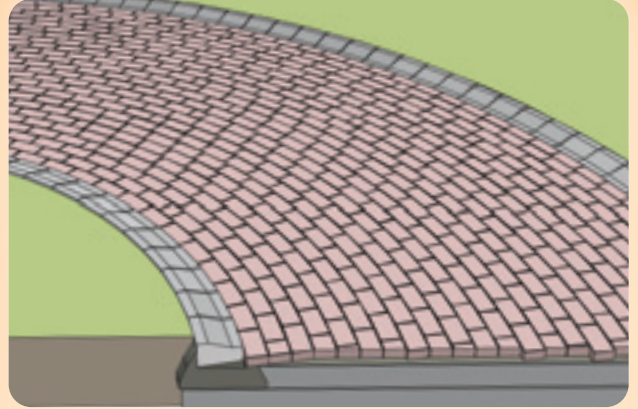
ÍVES ÚT "K" SZEGÉLLEL, HOSSZANTI FEKTETÉSSEL
