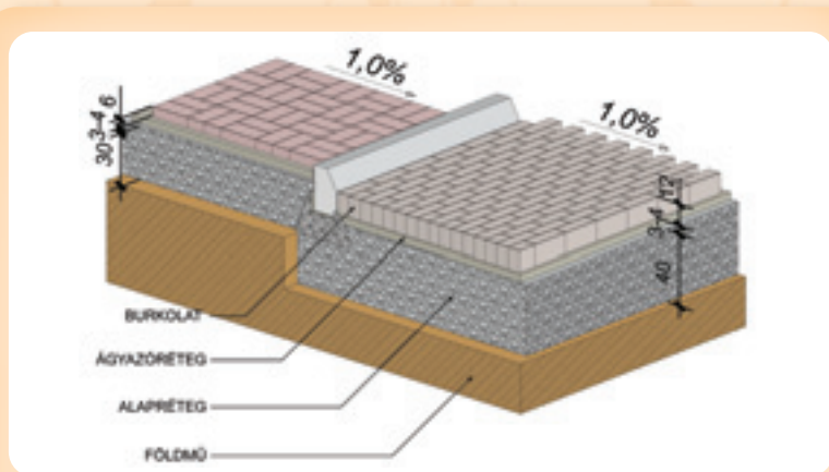
6 CM-ES TÉGLAKÓ TÖMB KÖTÉSBEN, KIEMELT SZEGÉLLEL ÉS ÁLLÍTOTT 8 CM-ES TÉGLAKÓ FUTÓSOROS MINTÁVAL
