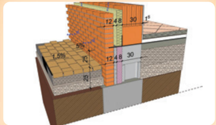
KISZELLŐZTETETT HOMLOKZATI TÉGLAKŐ BURKOLAT PERSPEKTIVIKUS KÉPE
