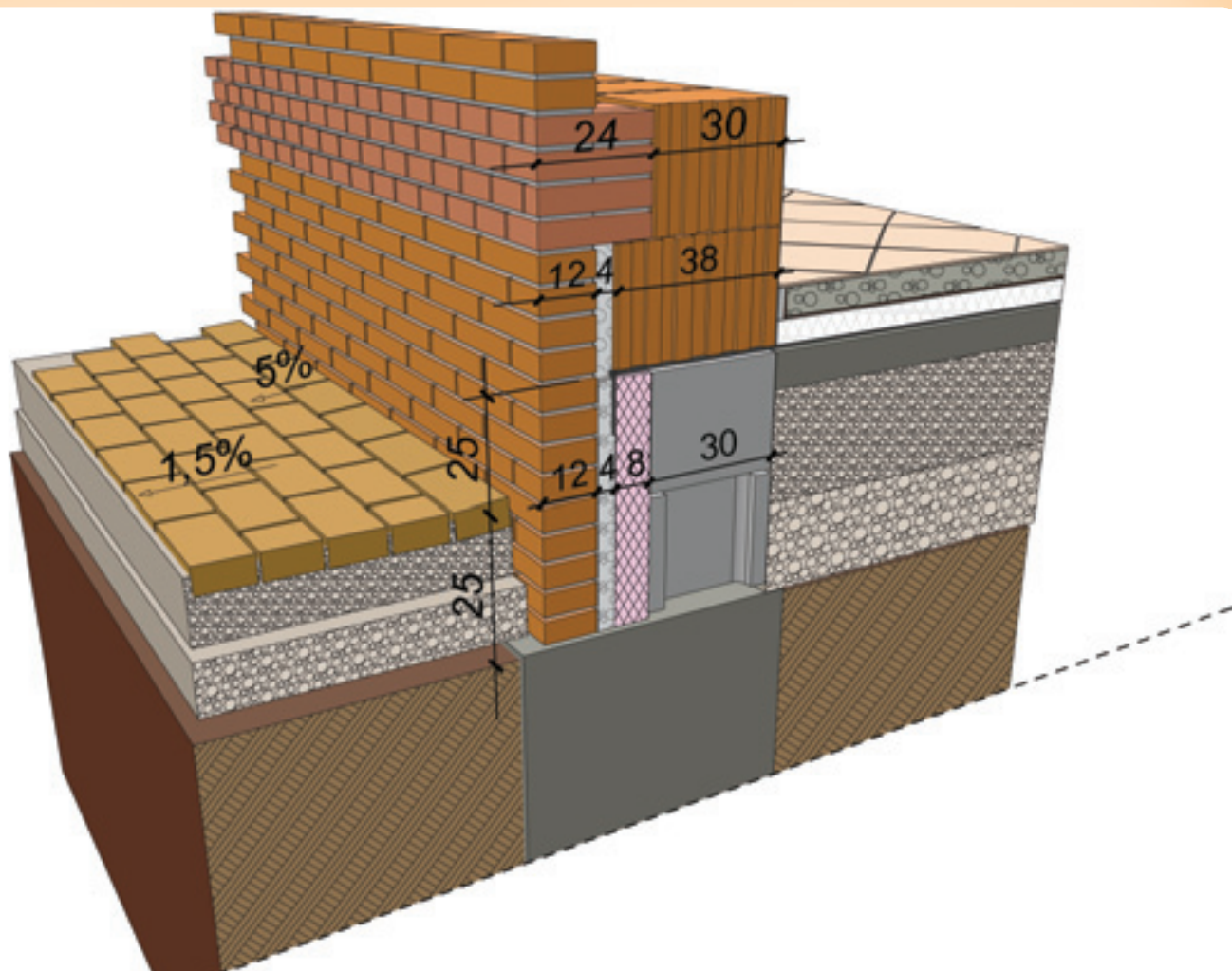
EGYBEFALAZOTT HOMLOKZATI TÉGLAKŐ BURKOLAT PERSPEKTIVIKUS KÉPE
