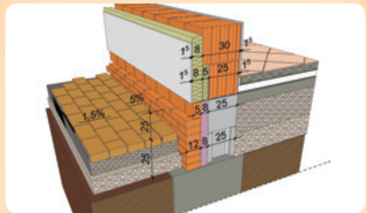
FEKVŐSOROS TÉGLAKŐ LÁBAZAT PERSPEKTIVIKUS KÉPE
