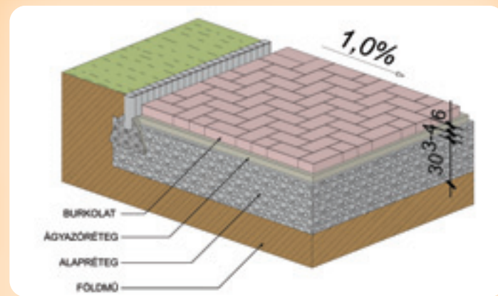
JÁRDAKŐ BURKOLAT SORSZEGÉLLEL HALSZÁLKA MINTÁVAL
