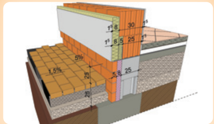
ÁLLÓSoros TÉGLAKŐ LÁBAZAT PERSPEKTIVIKUS KÉPE
