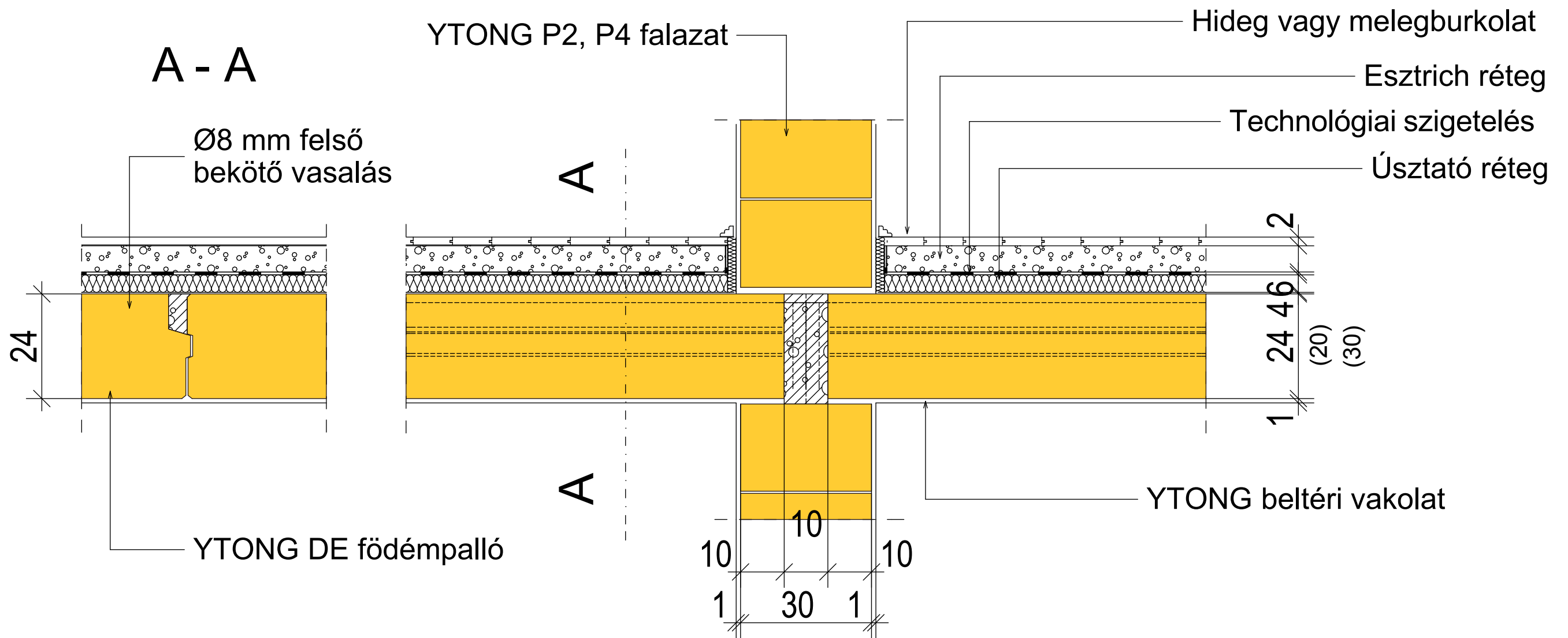
hosszmetszet
