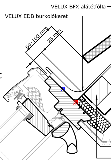
A-A metszet 1:5
